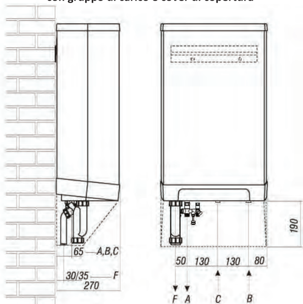
Dimensioni d'ingombro generatore termico con gruppo di carico e cover di copertura
