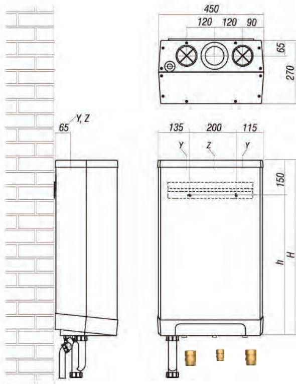
Dimensioni d'ingombro generatore termico
