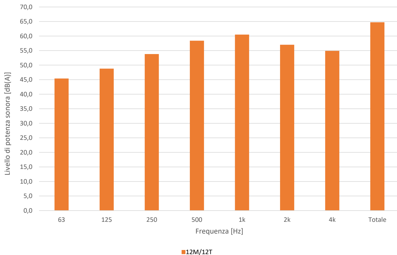
Livello di potenza sonora Lw unità 12M/12T [dB(A)]
