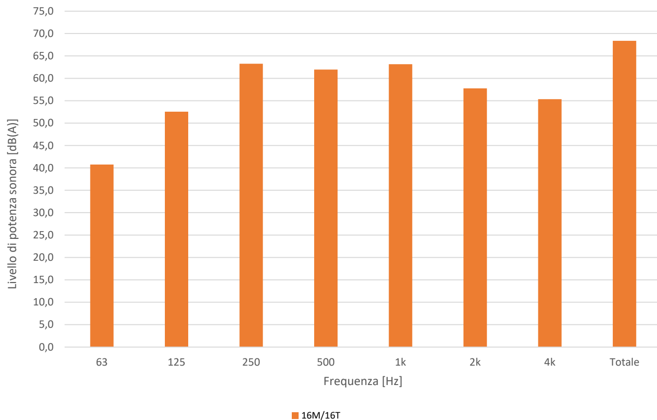
Livello di potenza sonora Lw unità 16M/16T [dB(A)]
