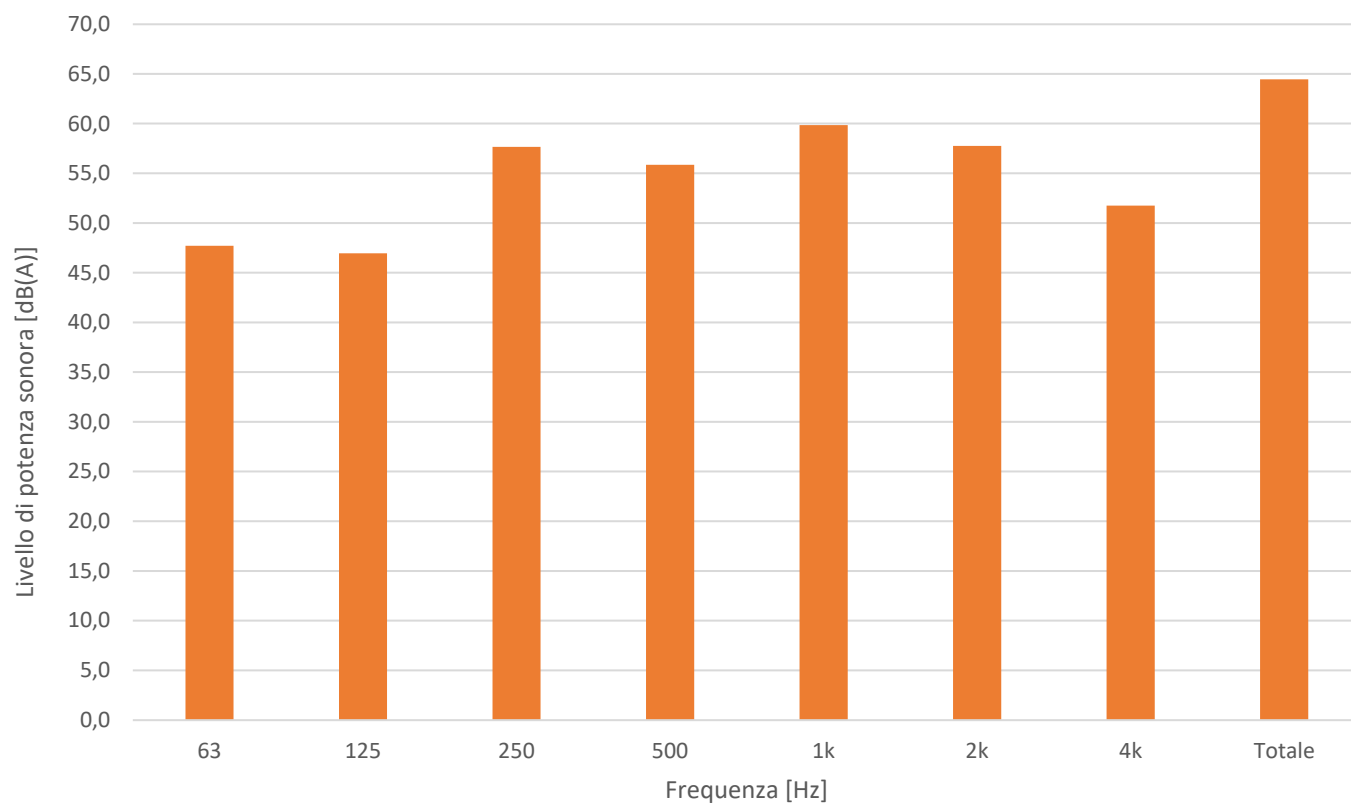
Livello di potenza sonora Lw unità 08A [dB(A)]
