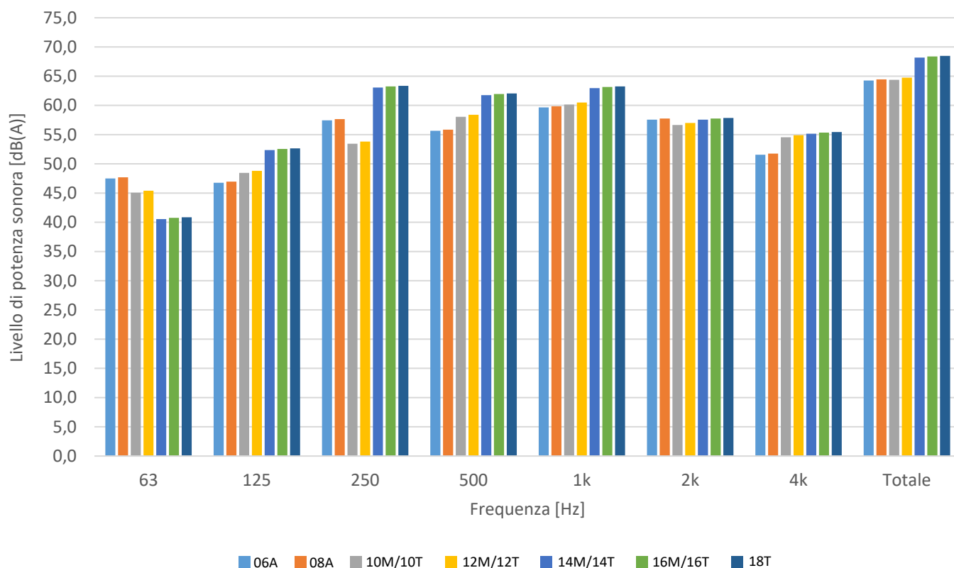
Livello di potenza sonora Lw unità standard [dB(A)]
