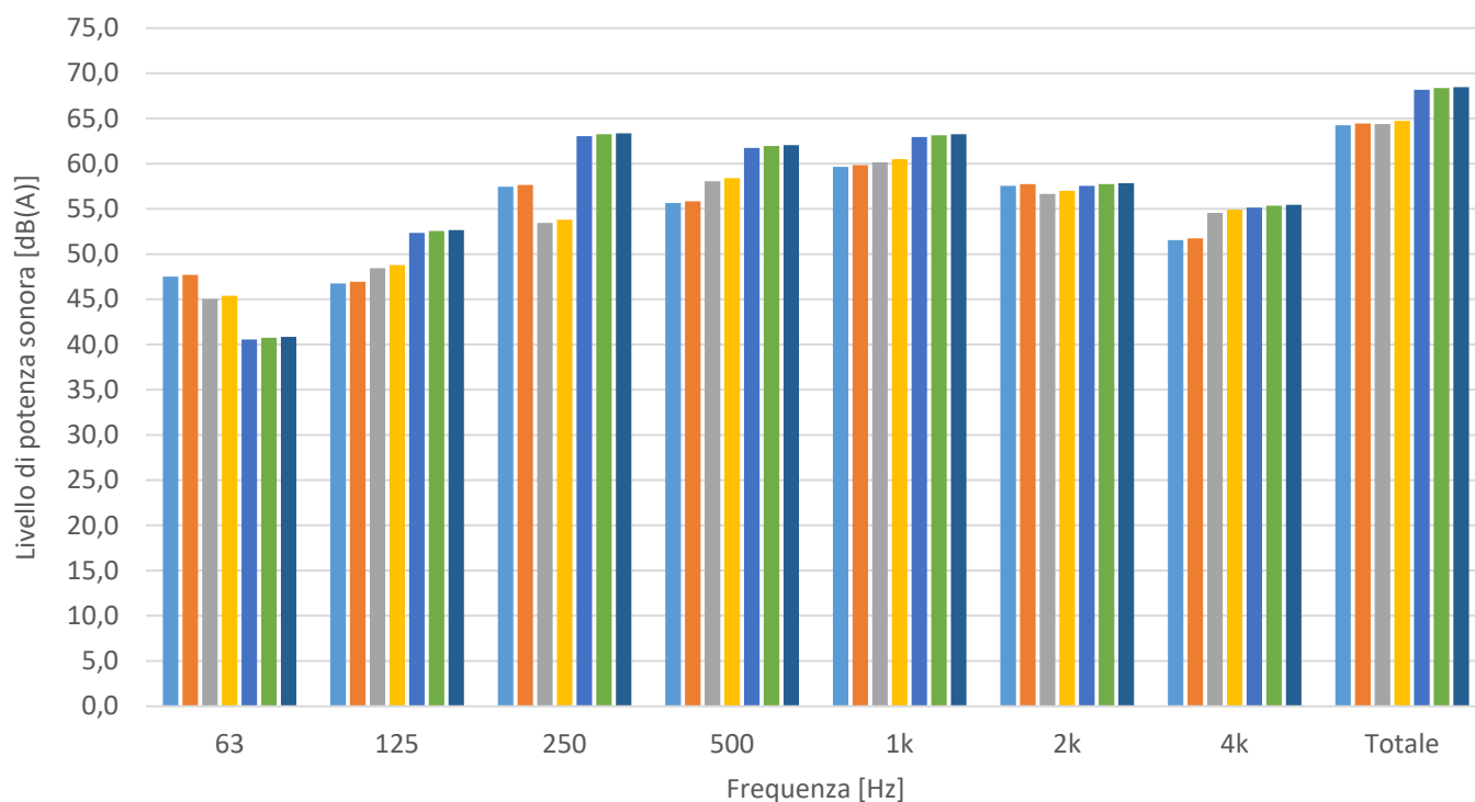
Livello di potenza sonora Lw unità standard [dB(A)]
